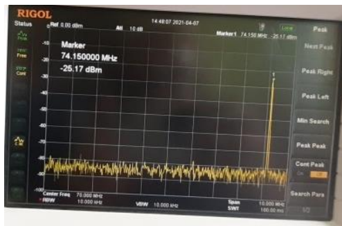
Рис. 4 – Выходной сигнал при V_T = 1,25 В
