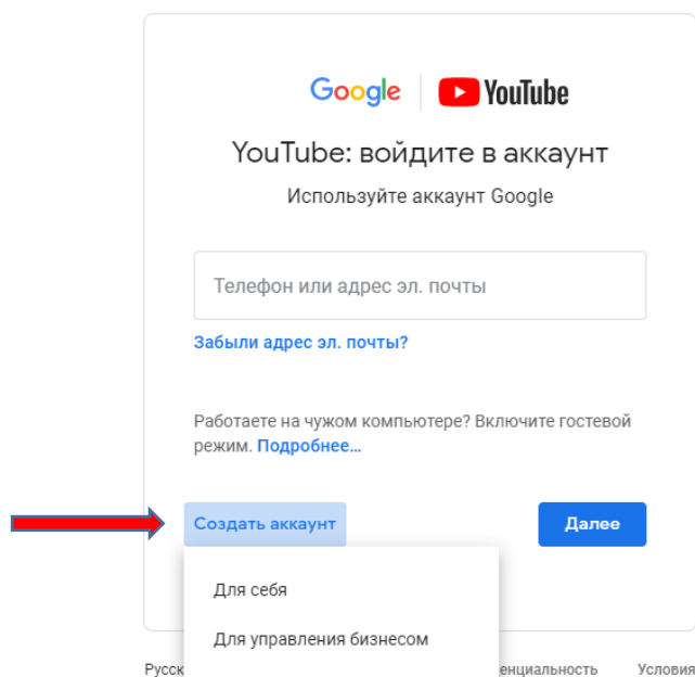
Рис.2 Регистрация
