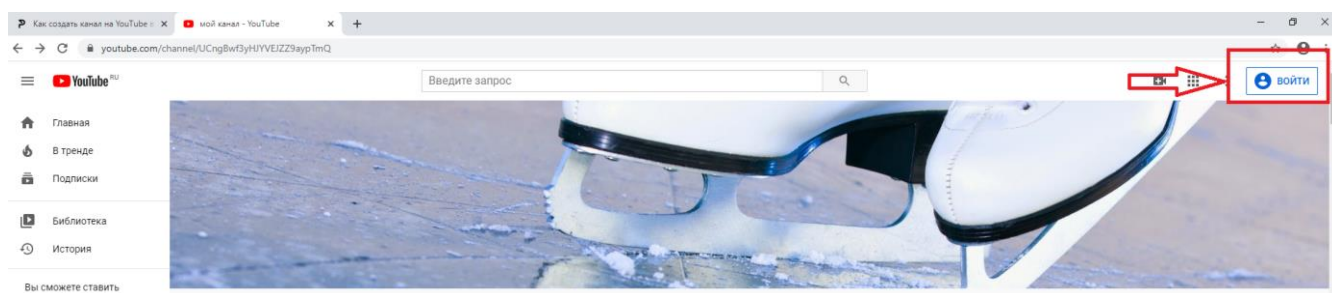
Рис. 1 Главная страница
